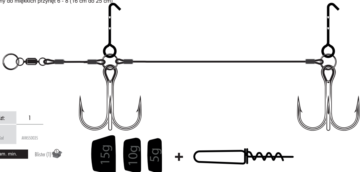
Skala 1:1
