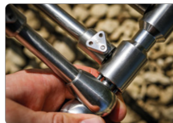
System blokady sprężynowej Dutch Pin.
