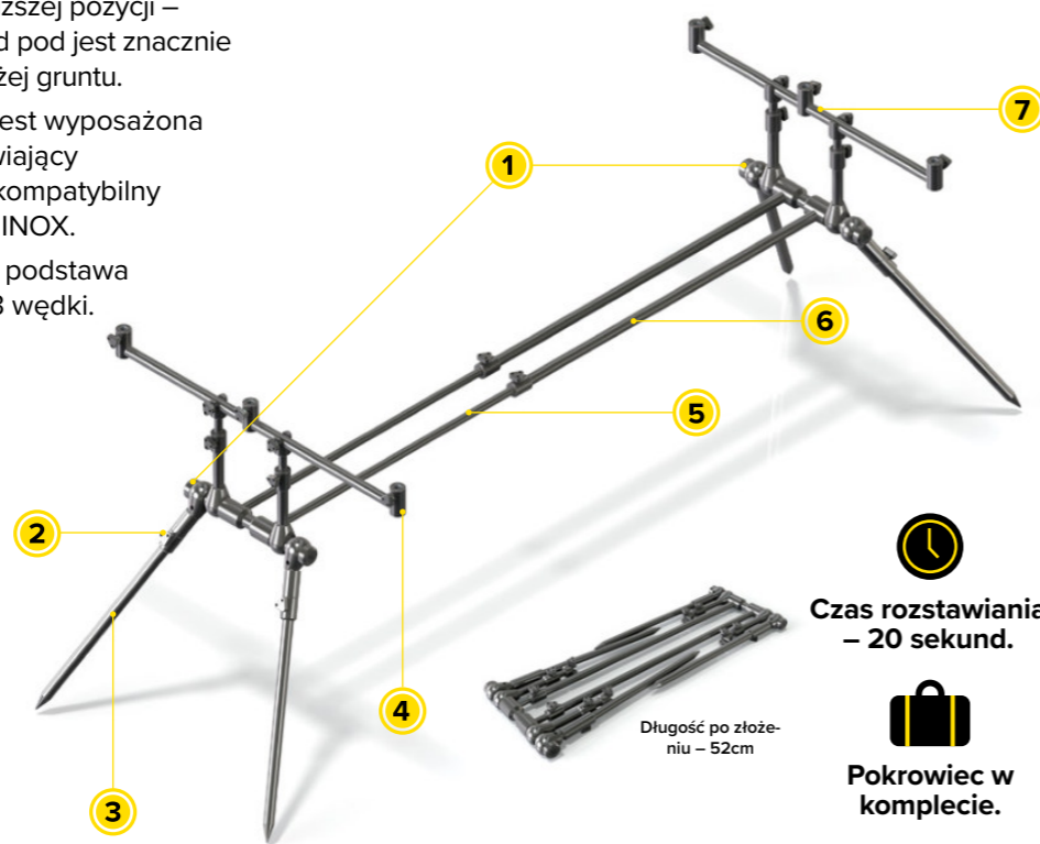
System blokady sprężynowej Dutch Pin.
